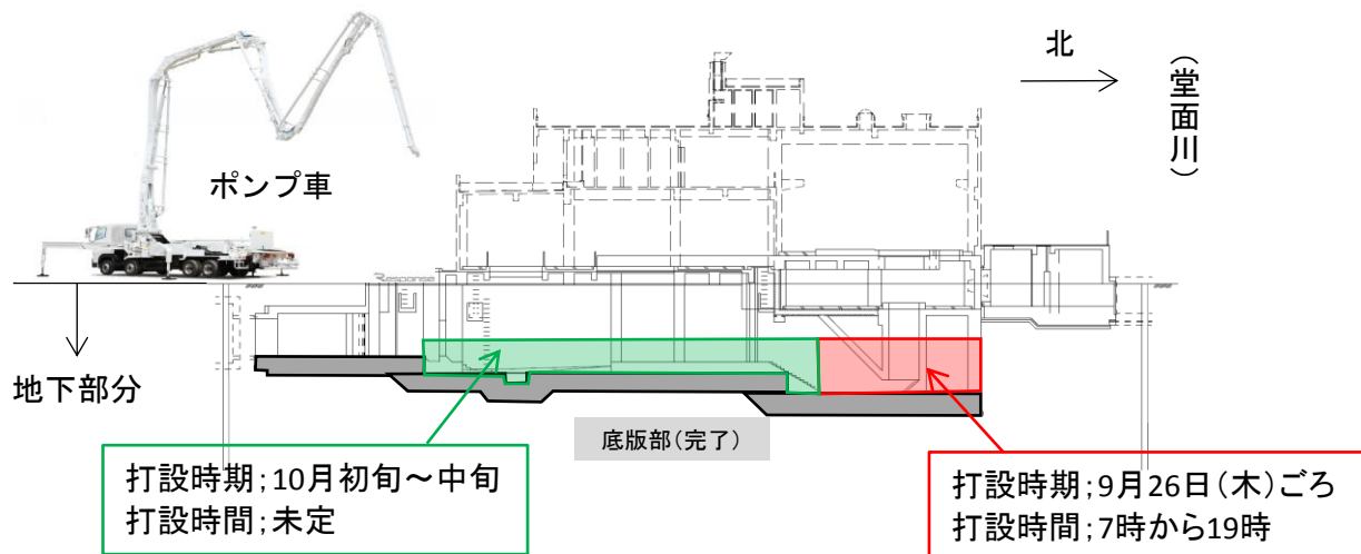
コンクリート打設時期、作業時間
