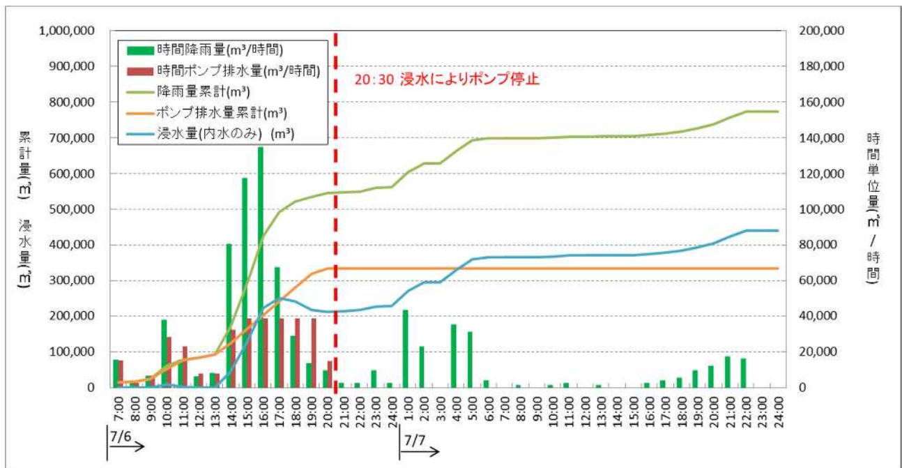
図 5-3-14 三川排水区における流入-流出グラフ
