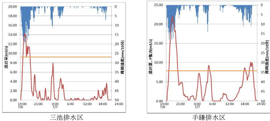
図 5-3-16 各排水区におけるハイドログラフによる浸水想定（その2）
