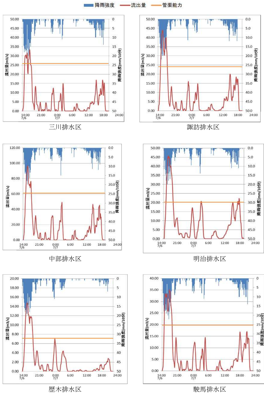
図 5-3-15 各排水区におけるハイドログラフによる浸水想定（その 1）
