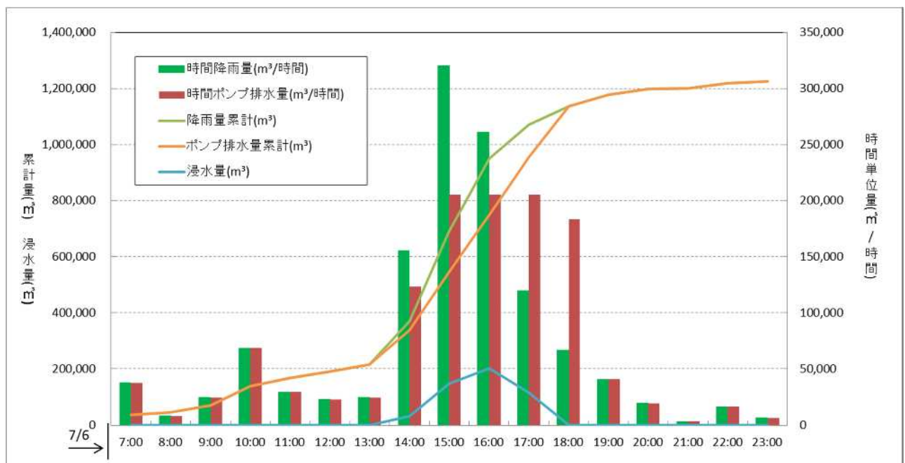
図 5-3-11 中部排水区における流入-流出グラフ
