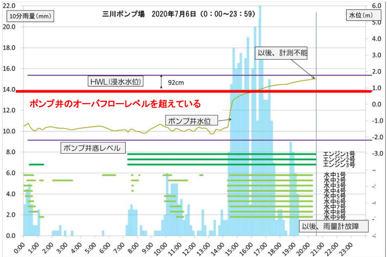
図 5-3-6 三川ポンプ場における災害時の状況(稼働状況、水位、降雨状況)
