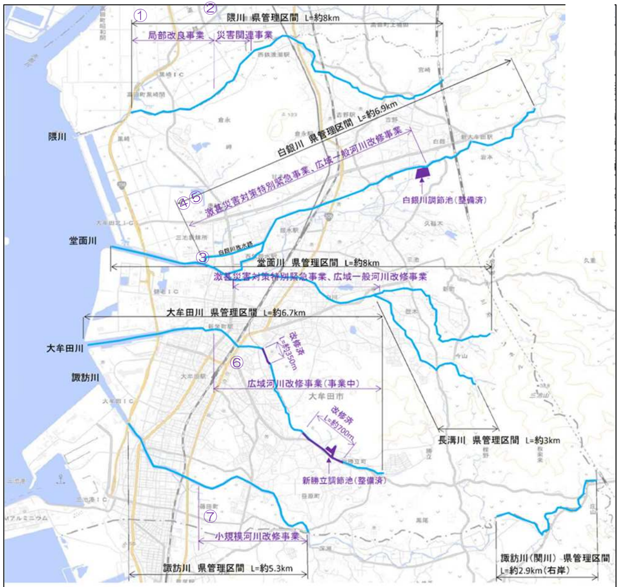
図 5-3-2 二級河川の整備状況図
