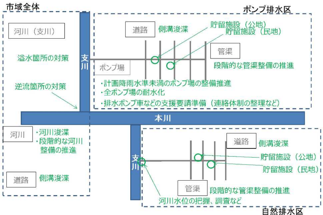
図 参考-2-1 排水対策基本計画の対策概要図
