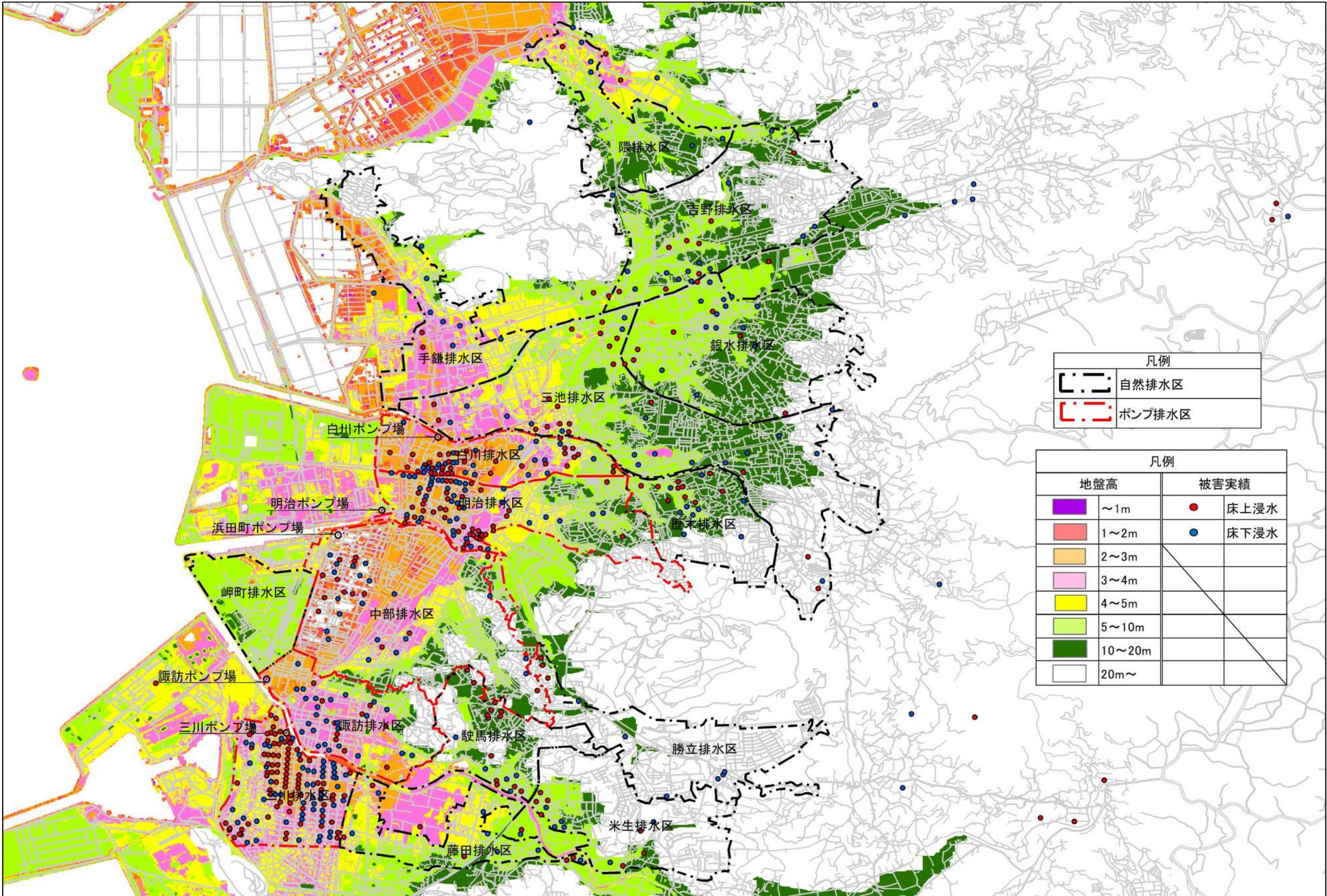
図 5-3-22 浸水被害箇所(床上、床下浸水)と地盤高の重ね合わせ
