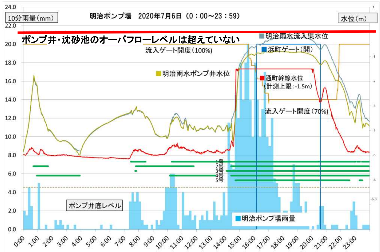
図 5-3-4 明治ポンプ場における災害時の状況(稼働状況、水位、降雨状況)
