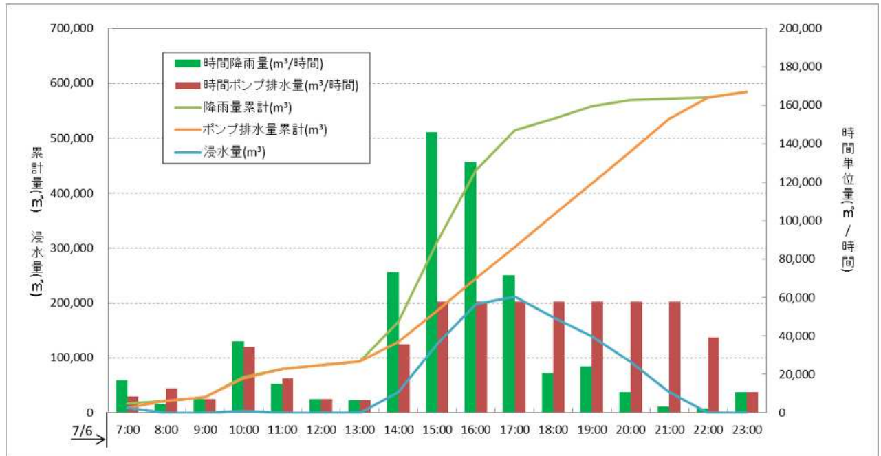
図 5-3-13 諏訪排水区における流入-流出グラフ
