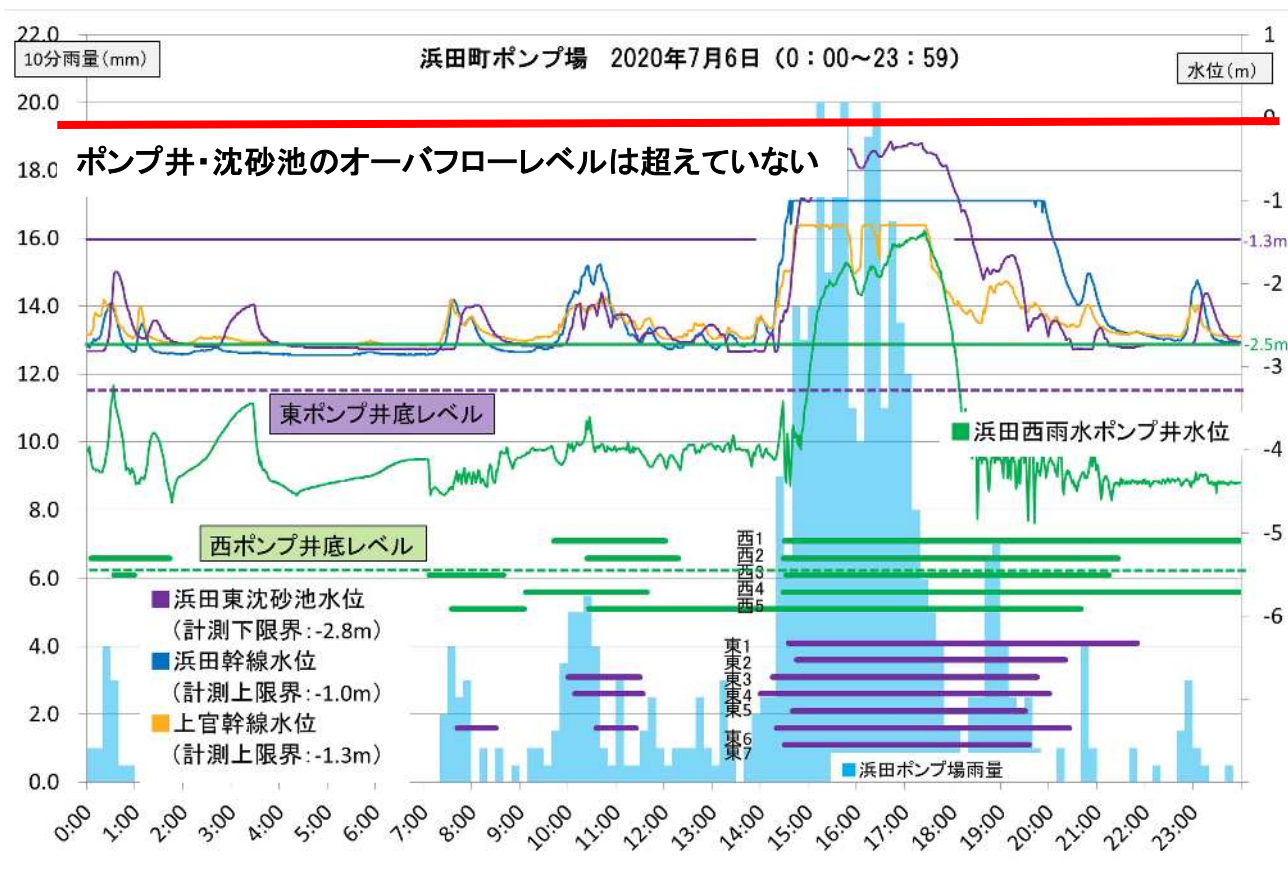
図 5-3-3 浜田町ポンプ場における災害時の状況(稼働状況、水位、降雨状況)
