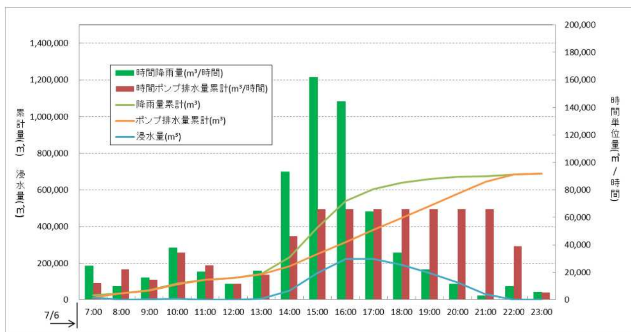
図 5-3-12 明治排水区における流入-流出グラフ
