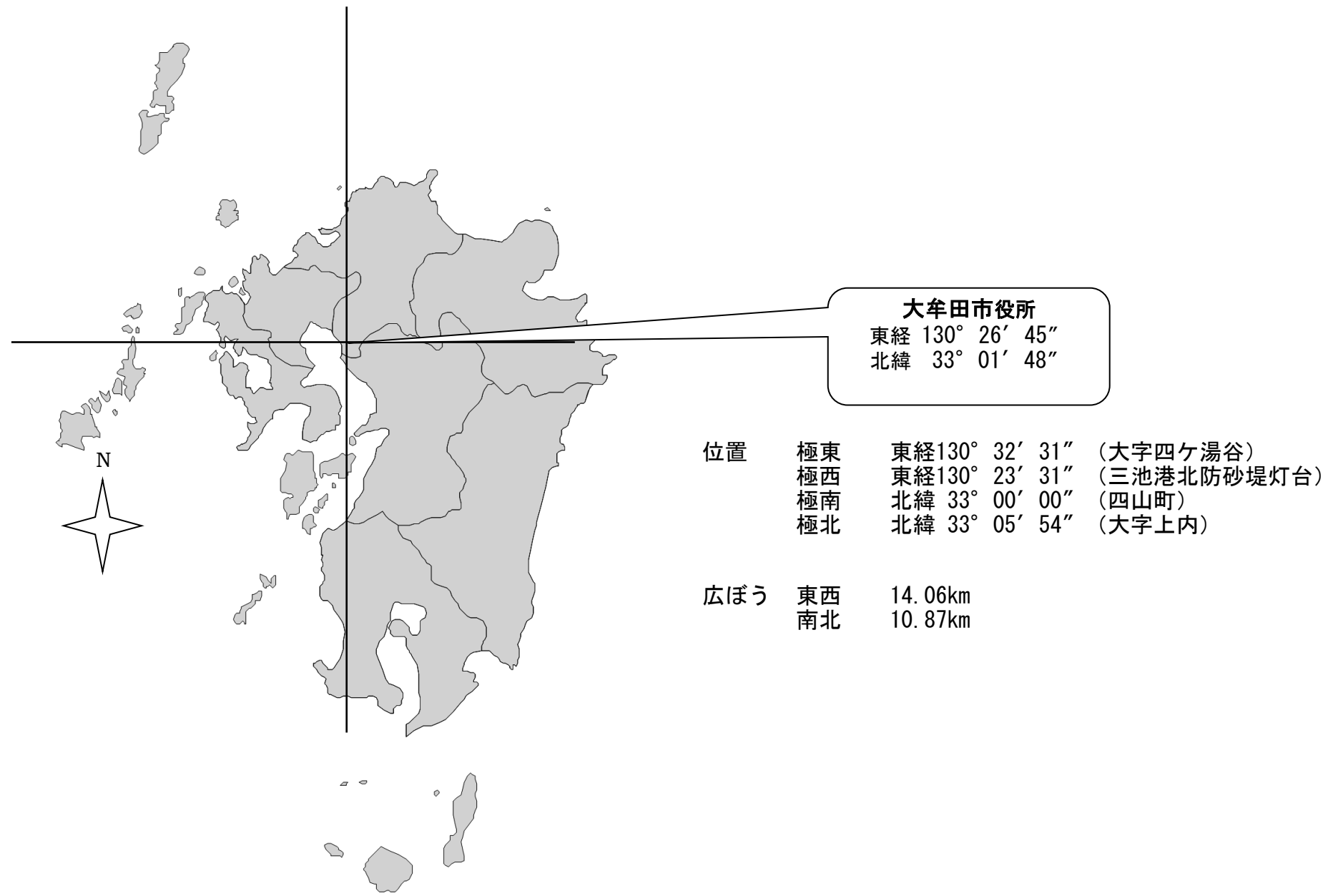
大牟田市の位置（平成29年4月1日現在）
