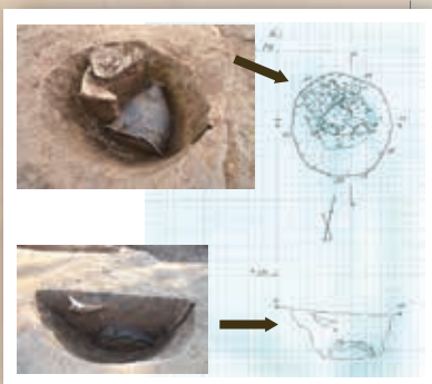
遺構の実測図（土坑を真上から見た図） 写真と断面を真横から見た図・写真。 穴の中に土器があります。
