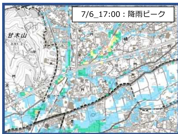
図 2.2.22 橘・吉野などの地区の浸水状況（浸水シミュレーション：令和2年7月豪雨）
