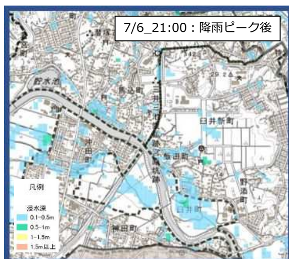
図 2.2.10 臼井町・飯田町・馬込町などの地区の浸水状況（浸水シミュレーション：令和2年7月豪雨）
