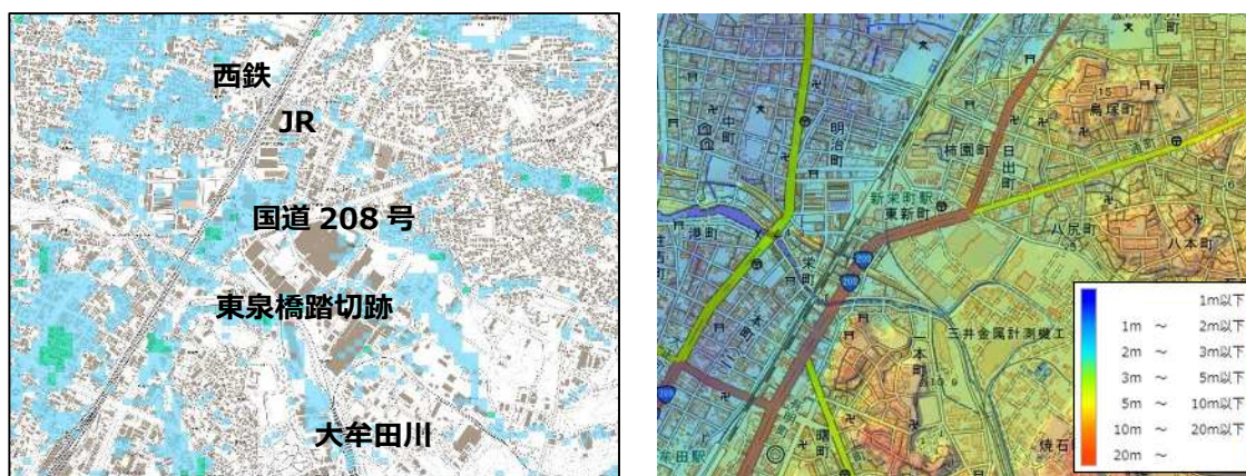
図 2.2.11 旭町地区の浸水解析結果と地形・地盤高
