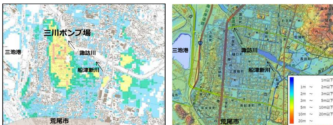
図 2.2.5 三川地区の浸水解析結果と地形・地盤高
