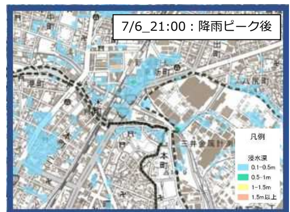
図 2.2.12 旭町地区の浸水状況 (浸水シミュレーション：令和2年7月豪雨)
