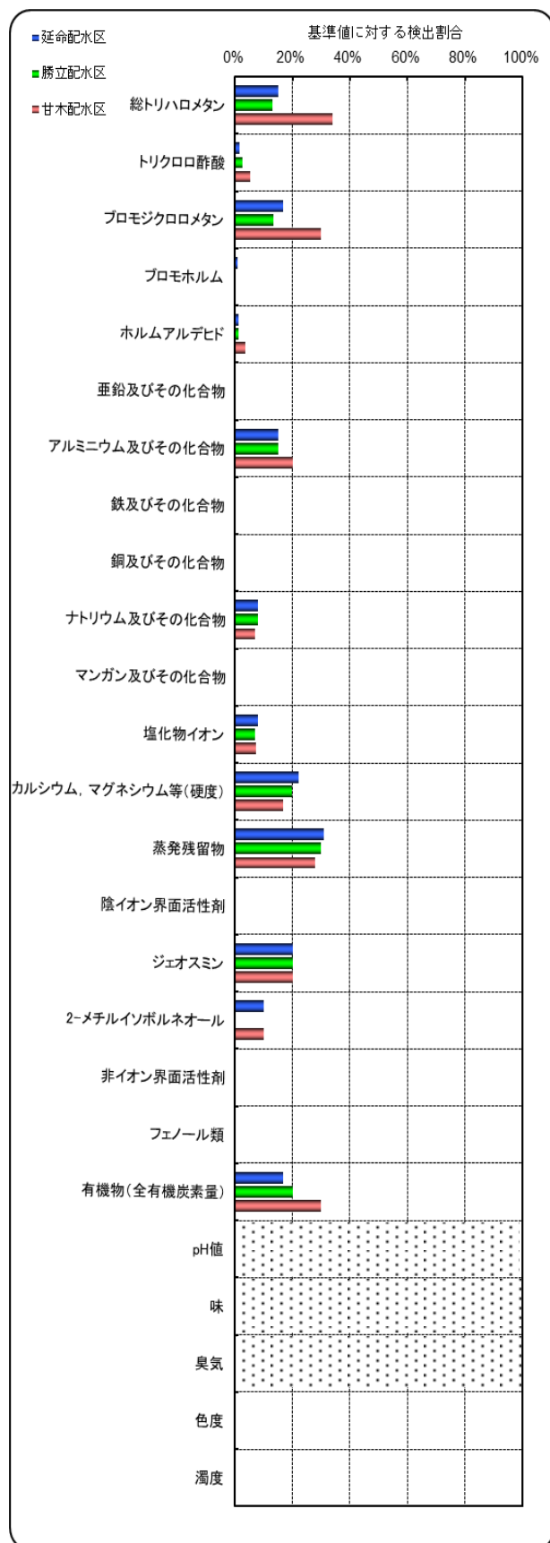
図2 各配水系統において検出された年間最高値の基準値に対する割合(令和3年度)
