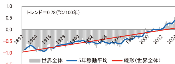
世界の年平均気温へん差
