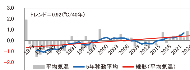
大牟田の年平均気温へん差
