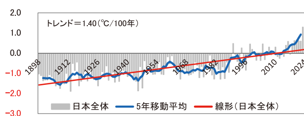
日本の年平均気温へん差
