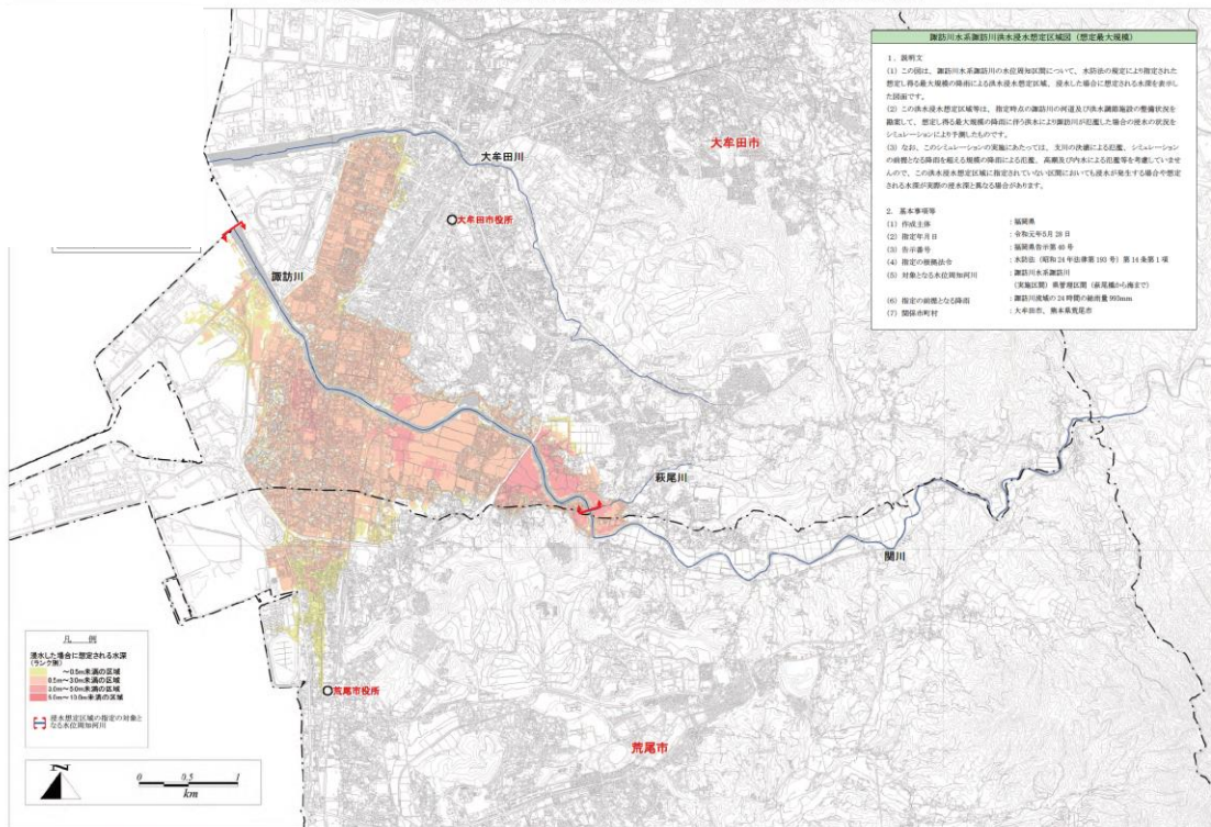
諏訪川水系諏訪川洪水浸水想定区域図（想定最大規模）
