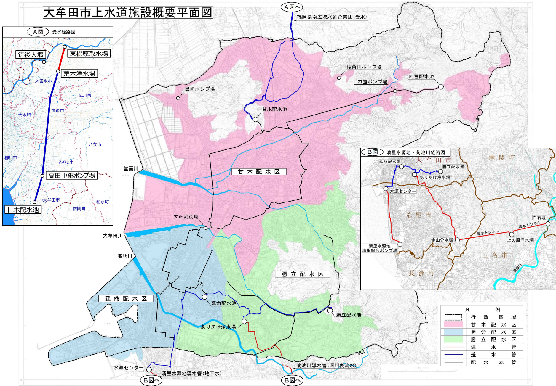
図 2-2 大牟田市上水道施設概要平面図
