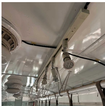
客席側配線・レール
