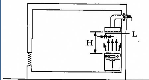
V=30kQ (ハ) 排気フードⅠ型 H: 1m以下 L: H/10以上
