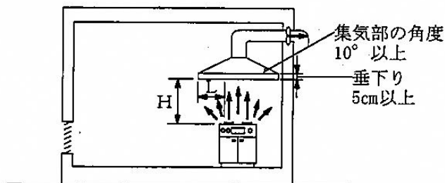
V=20kQ (ニ) 排気フードⅡ型 H: 1m以下 L: H/2以上
