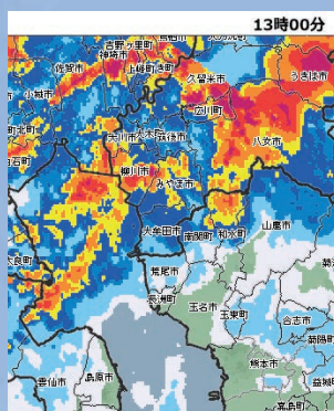
令和2年7月6日の雨雲レーダーの様子
